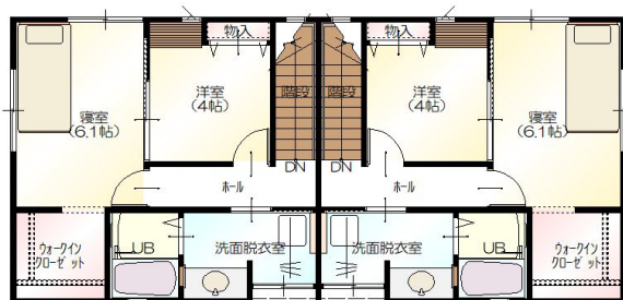
2F
